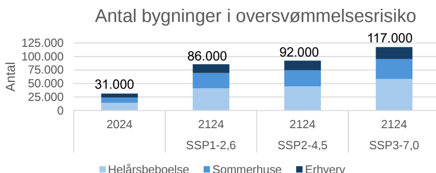
Figur 6: Antal helårsboliger, erhvervsbygninger og sommerhuse som er truet af oversvømmelser fra stormfloder i Danmark i dag (2024) og i år 2124 for klimascenarierne SSP1-2,6, SSP2-4,5 og SSP3-7,0.
