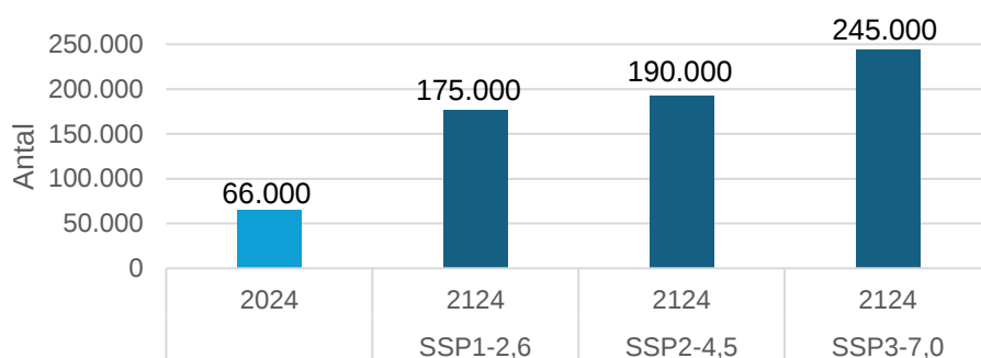
Figur 4: Antal personer som bor i ejendomme som er truet af oversvømmelser fra stormfloder i Danmark i dag (2024) og i år 2124 for klimascenarierne SSP1-2,6, SS2-4,5 og SSP3-7,0.
