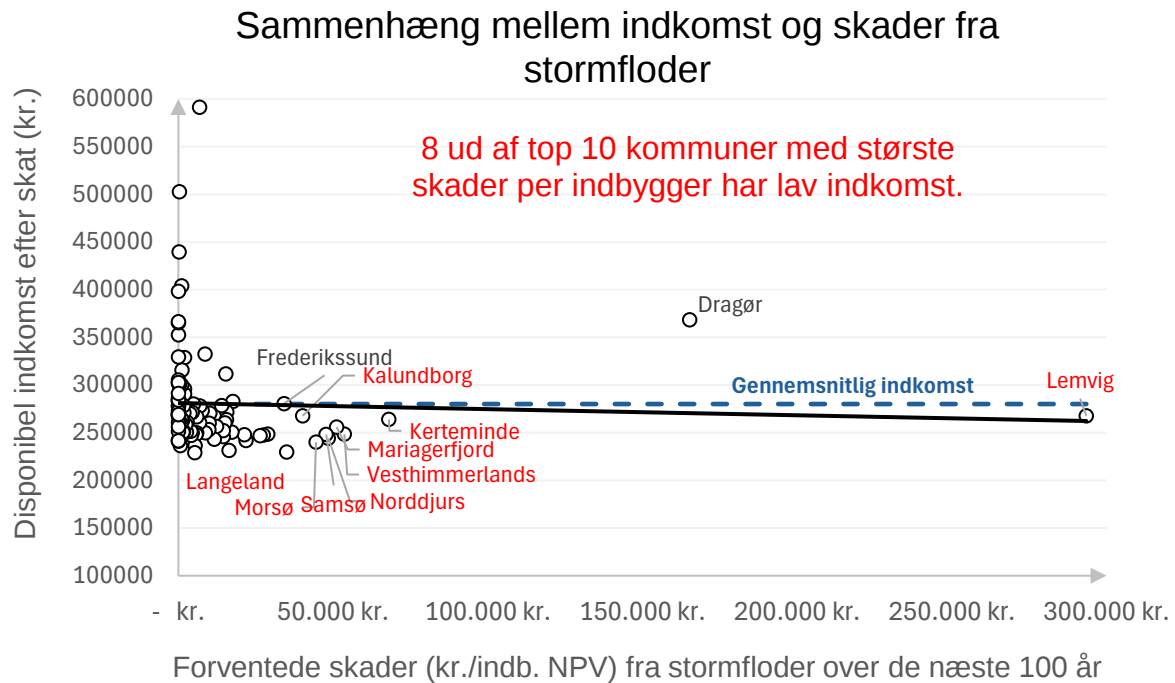
Figur 3: Sammenhæng mellem disponibel indkomst og skade for helårsboliger per indbygger ved stormfloder i perioden 2024-2124 for scenarie SSP2-4,5 på kommuneniveau.
