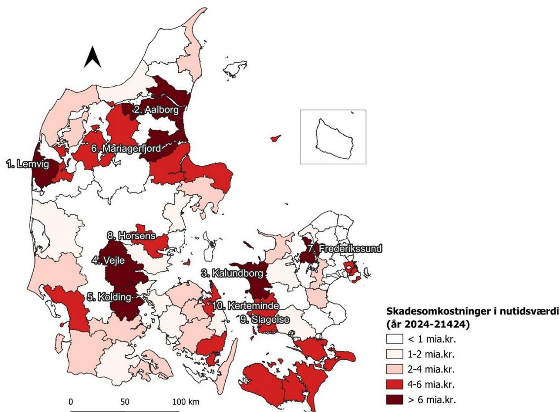
Figur 2: Forventede skader i nutidsværdi for oversvømmelser fra stormflod over de næste 100 år (år 2024-2124), fordelt på kommuneniveau for klimascenariet SSP2-4,5. Værdierne 1-10 angiver kommuner med størst omkostninger.
